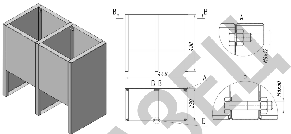
Рисунок 1 - Подставка напольная ПРЕСТИЖ под 2 огнетушителя
