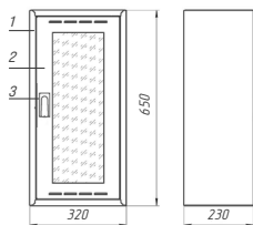
Рисунок 1- Шкаф пожарный ПРЕСТИЖ-04
